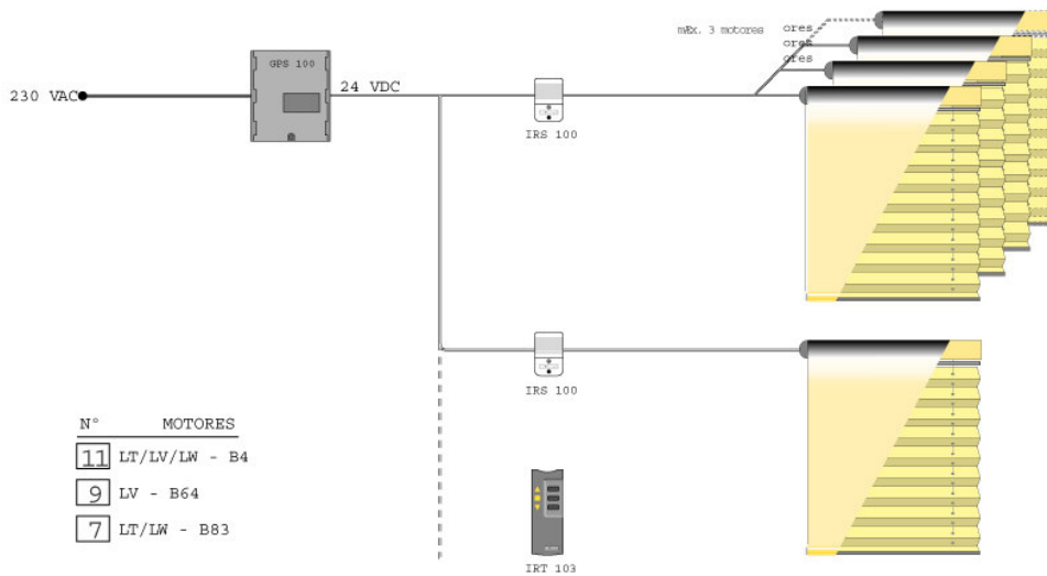
GPS 100 - 2 x IRS 100 - IRT 103
