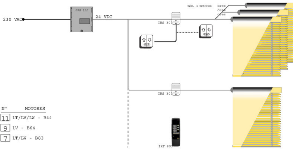
GPS 100 - 2 x IRS 300 - IRT 803
