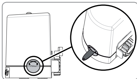
Motor bloqueado
